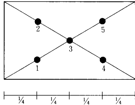
煙排出口の風速測定位置
