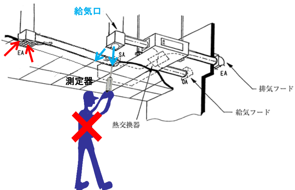
二酸化炭素の含有率の測定 (悪い例)
