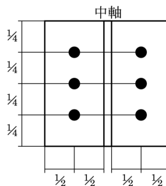
排煙口の風速測定位置
