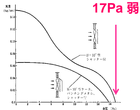
換気扇（圧力扇）の風量特性の例
